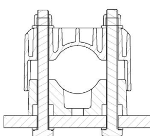
Zwillingsbefestigung
