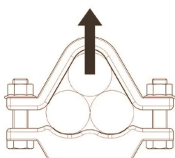
CHARGE LATÉRALE DIRECTION 'VERTICALE'
