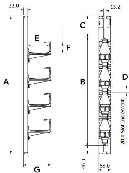
CC01 Hanger
