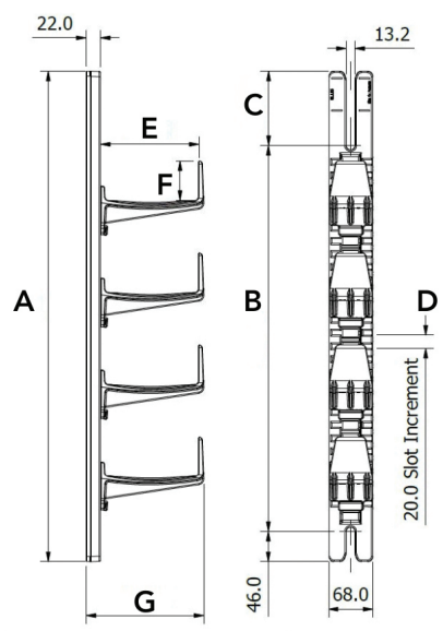
CC02 Hanger
